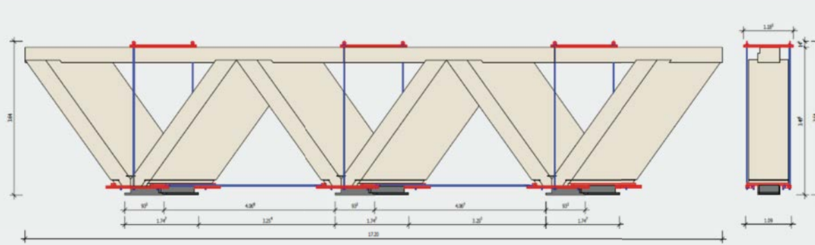
Die Zeichnung zeigt die Lage und die Angriffspunkte der Stahl-Hebe-Konstruktion am Fachwerk-Fassadenelement.
